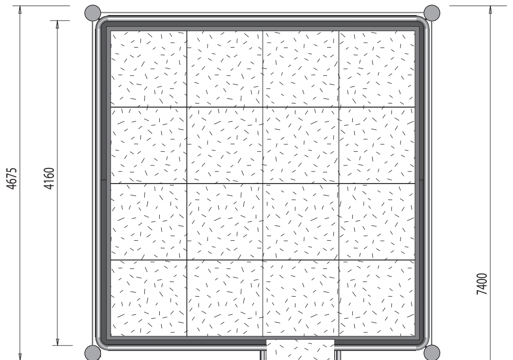
Draufsicht - Balkonturm Grundriss
