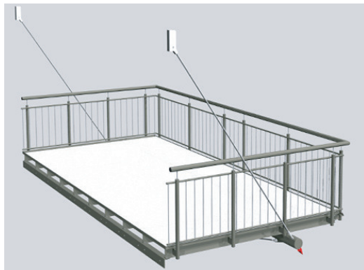
Abbildung: HÄNGE-BALKON Auskrägung 2895mm Breite 5600mm Geländer Staketten Konstruktion Aluminium in Grau DB 703 pulverbeschichtet Unterspannung 3 Feld Balkonbelag Alu-Riffelblech Duett in "Weiß Marmor Feinstruktur" pulverbeschichtet.
