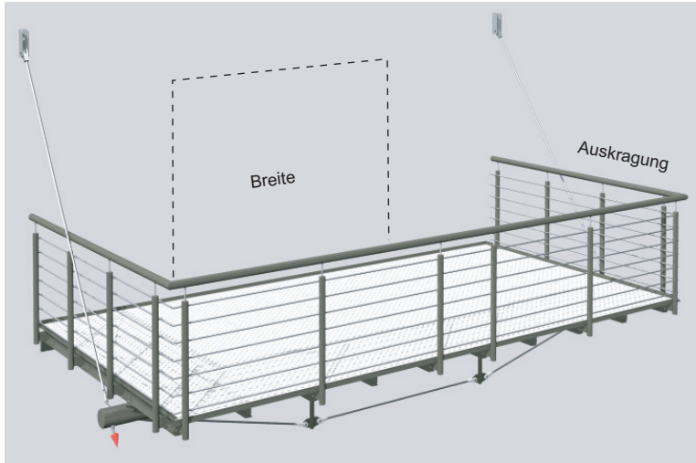
Abbildung: HÄNGE-BALKON Auskrägung 2895mm Breite 5600mm Geländer Reling Konstruktion Aluminium in Grau DB 703 pulverbeschichtet Unterspannung 3 Feld Balkonbelag Alu-Riffelblech Duett in "Weiß Marmor Feinstruktur" pulverbeschichtet.
