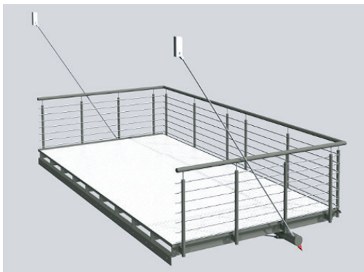
Abbildung: HÄNGE-BALKON Auskrägung 2895mm Breite 5600mm Geländer Reling Konstruktion Aluminium in Grau DB 703 pulverbeschichtet Unterspannung 3 Feld Balkonbelag Alu-Riffelblech Duett in "Weiß Marmor Feinstruktur" pulverbeschichtet.
