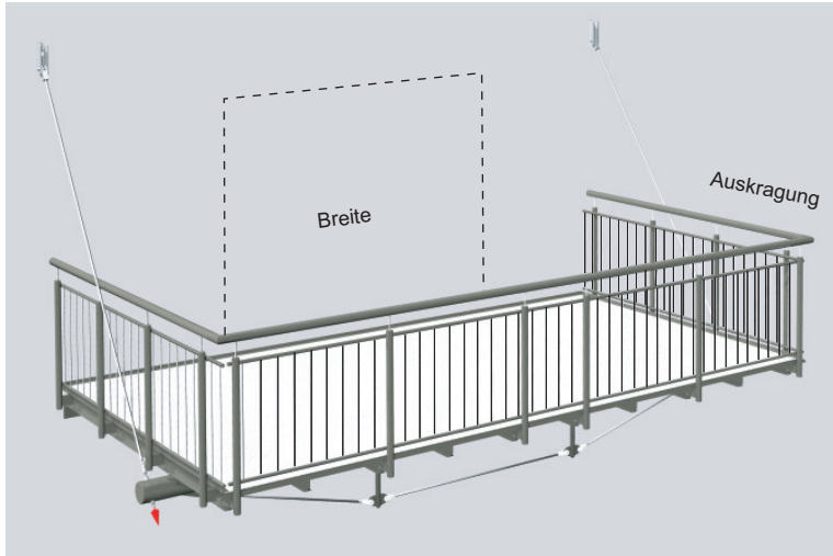
Abbildung: HÄNGE-BALKON Auskrägung 2895mm Breite 5600mm Geländer Staketten Konstruktion Aluminium in Grau DB 703 pulverbeschichtet Unterspannung 3 Feld Balkonbelag Alu-Riffelblech Duett in "Weiß Marmor Feinstruktur" pulverbeschichtet.
