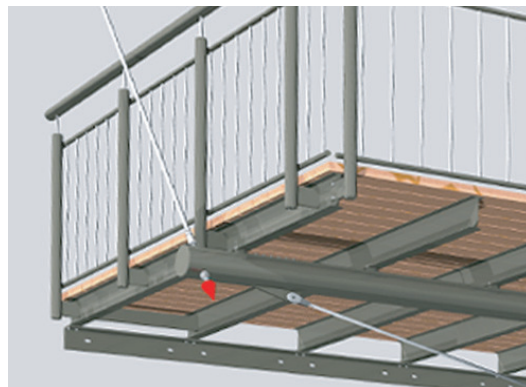
Abbildung: HÄNGE-BALKON Auskrugung 2895mm Breite 5600mm HB-AL-DGA 07-06 Geländer Staketten Konstruktion Aluminium in Grau DB 703 pulverbeschichtet Unterspannung 3 Feld Balkonbelag Douglasie Dielen geölt.
