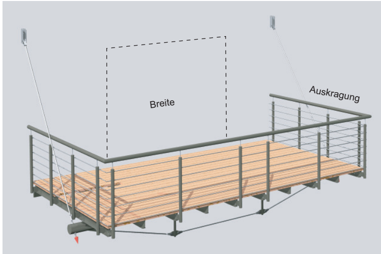
Abbildung: HÄNGE-BALKON Auskrugung 2895mm Breite 5600mm HB-AL-DGA 07-06 Geländer Reling Konstruktion Aluminium in Grau DB 703 pulverbeschichtet Unterspannung 3 Feld Balkonbelag Douglasie Dielen geölt.
