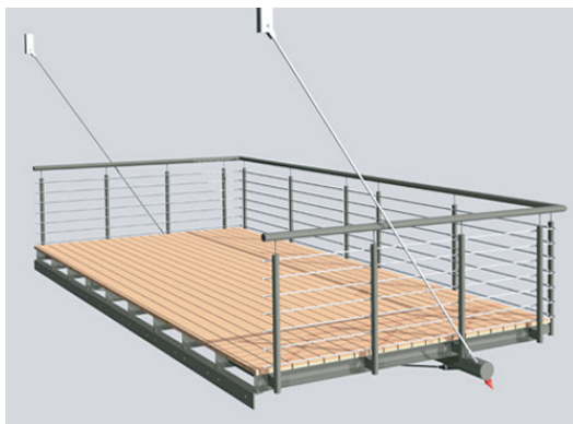
Abbildung: HÄNGE-BALKON Auskrugung 2895mm Breite 5600mm HB-AL-DGA 07-06 Geländer Reling Konstruktion Aluminium in Grau DB 703 pulverbeschichtet Unterspannung 3 Feld Balkonbelag Douglasie Dielen geölt.
