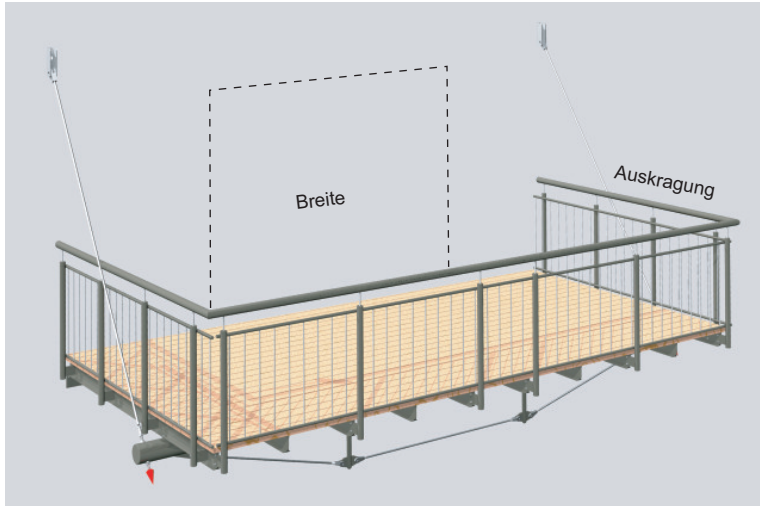
Abbildung: HÄNGE-BALKON Auskrugung 2895mm Breite 5600mm HB-AL-DGA 07-06 Geländer Staketten Konstruktion Aluminium in Grau DB 703 pulverbeschichtet Unterspannung 3 Feld Balkonbelag Douglasie Dielen geölt.
